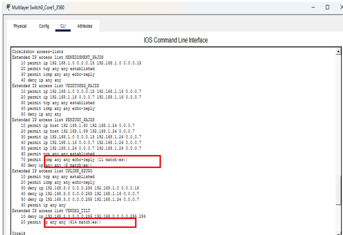
13. ábra ACL számlálók és találati statisztikák Forrás: Saját készítésű képernyőkép
