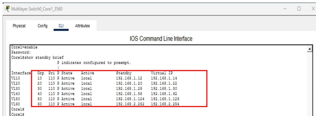
9. ábra HSRP állapot ellenőrzése a Core1 switchen. Forrás: Saját készítésű képernyőkép
