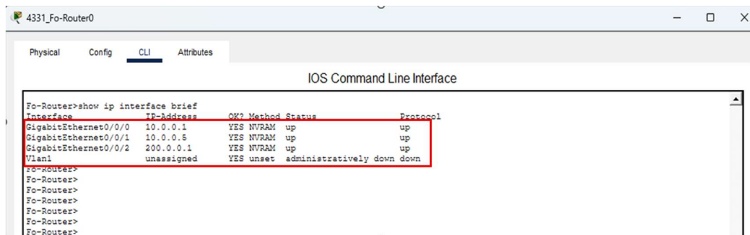
8. ábra Fő-Router interfészállapotainak ellenőrzése. Forrás: Saját készítésű képernyőkép
