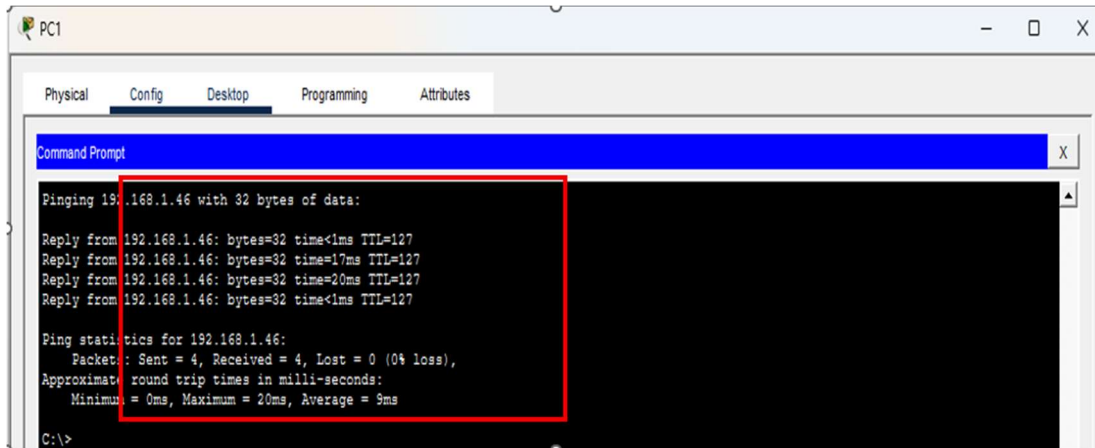
12. ábra PC1 → PC3 kommunikáció engedélyezése ACL segítségével Forrás: Saját készítésű képernyőkép
