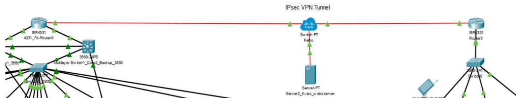
7. ábra Site to site VPN összeköttetés. Forrás: Saját készítésű képernyőkép
