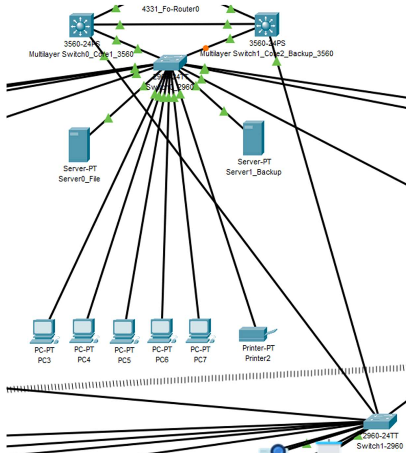
4. ábra Redundáns kábelezés core1-földszint sw, core2 földszint sw. Saját készítésű képernyőkép
