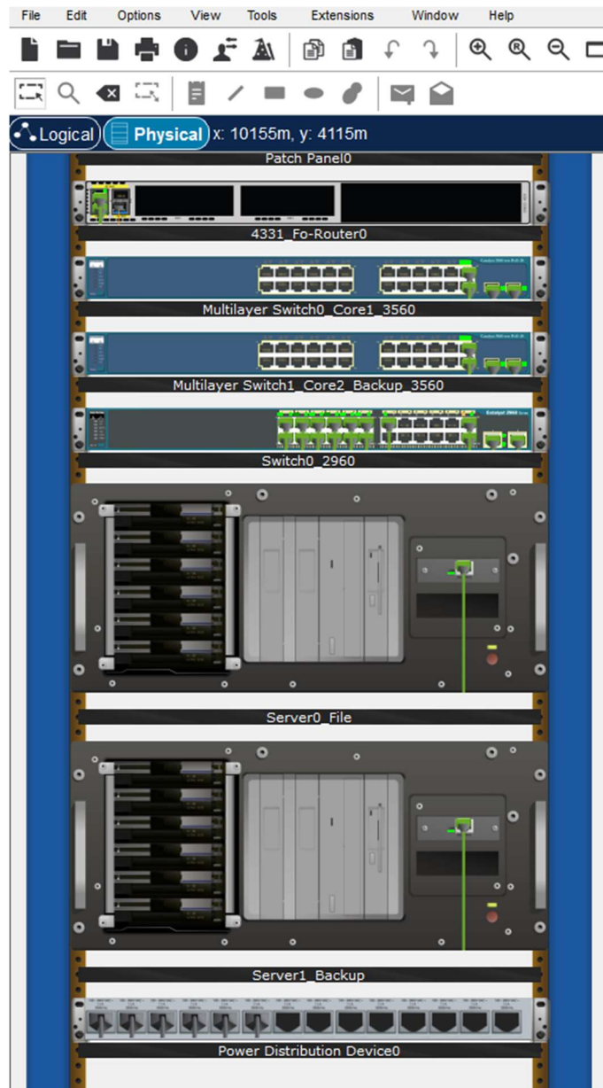
2. ábra Emeleti rack szekrény fizikai felépítése. Forrás: Saját készítésű képernyőkép
