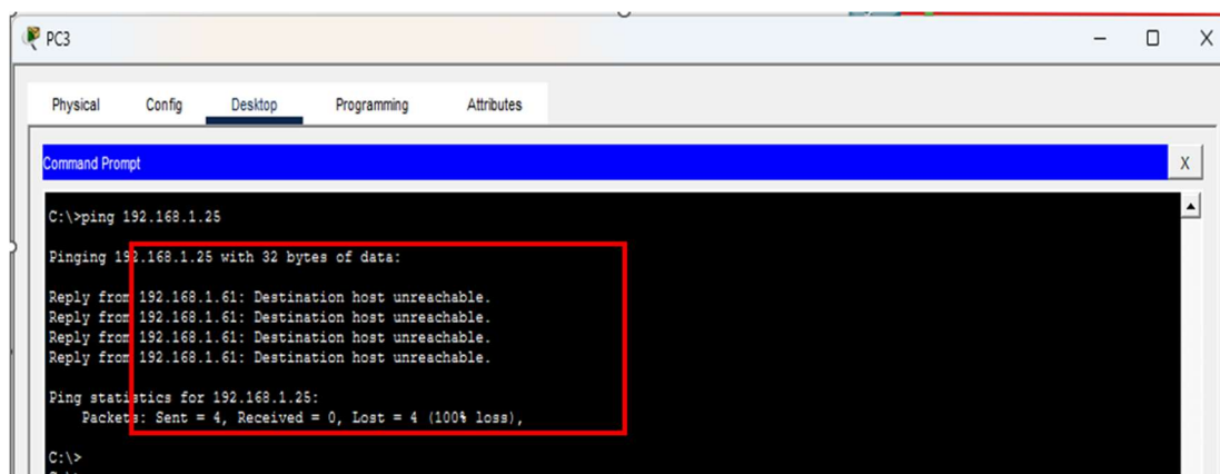
11. ábra PC3 → PC1 kommunikáció tiltása ACL segítségével Forrás: Saját készítésű képernyőkép
