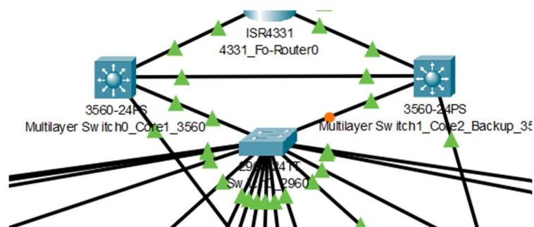
3. ábra Redundáns kábelezés core1-emelet sw, core2 emelet sw. Forrás: Saját készítésű képernyőkép
